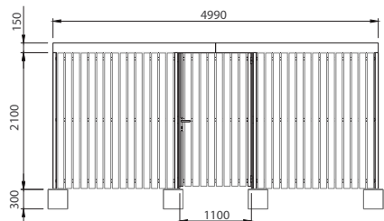
enkele deur breed 110cm
