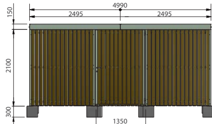
enkele deur breed 135cm
